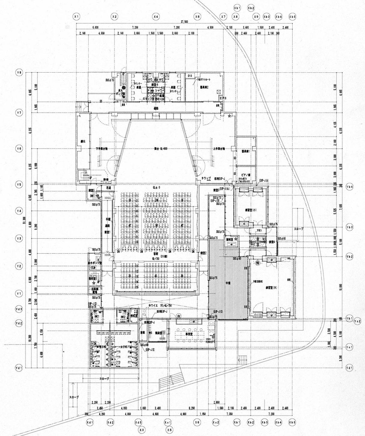
1階 平面図 1/200
