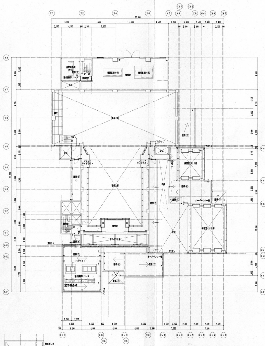
2階 平面図 1/200
