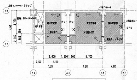
貯留庫・ピット 平面図 1/200
