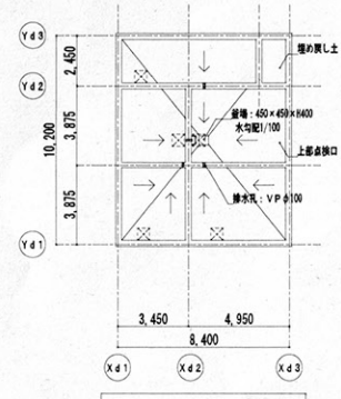
便所ピット 平面図 1/200
